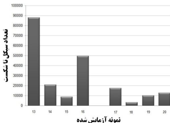
شکل ۷- پراکندگی تعداد سیکل تا شکست برای دسته دوم و سوم آزمایش خستگی
