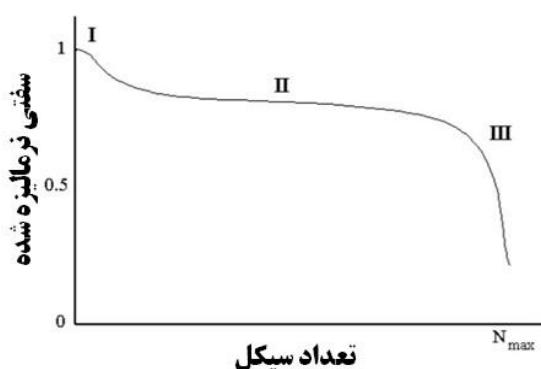
شکل ۱۰- مراحل افت سفتی در طی عمر خستگی
