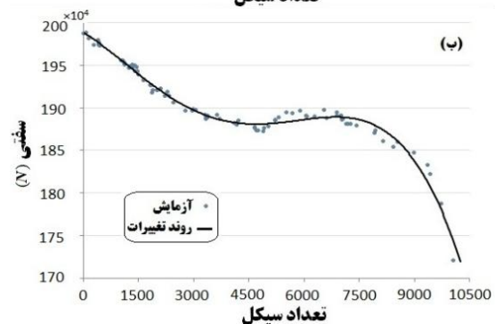
شکل ۱۱- افت سفتی در طی عمر خستگی: الف) نمونه آزمایشی شماره ۲ ( F_{max}=2200 \text{ N} ) و ب) نمونه آزمایشی شماره ۱۹ ( F_{max}=3000 \text{ N} )
