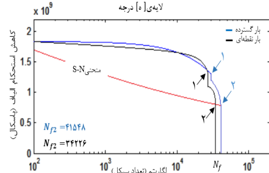
شکل ۶- نمودار محاسبه عمر خستگی گرافیت اپوکسی در مرحله دوم شکست
