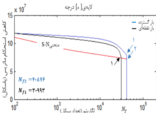
شکل ۱۰- نمودار محاسبه عمر خستگی شیشه اپوکسی در مرحله دوم شکست
