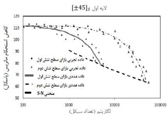
شکل ۴- نمودار صحت سنجی نتایج حل بدست آمده از روش عددی با استفاده از تئوری ساها و پروتمن با نتایج تجربی موجود در مرجع برای نمونه S45±
