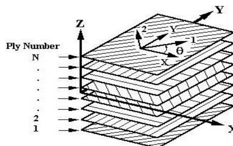
شکل ۲- چینش لایه‌ها در یک ورق چند لایه کامپوزیتی
