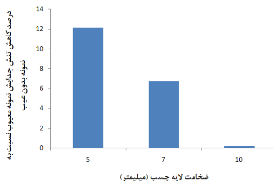
شکل ۱۰- نمودار درصد کاهش بار آغاز جدایش بر حسب ضخامت لایه چسب
