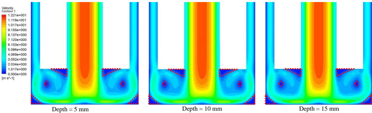
شکل ۸- کانتورهای سرعت
