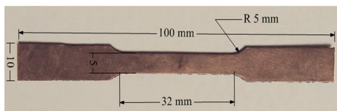
شکل ۱- ابعاد نمونه کشش استاندارد بر حسب میلی‌متر [۱۳]
