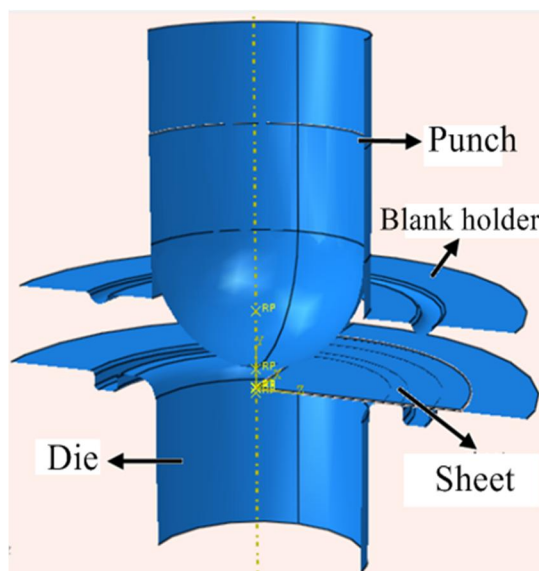
شکل ۷- شماتیک مدل‌سازی هندسی در نرم افزار آباکوس
