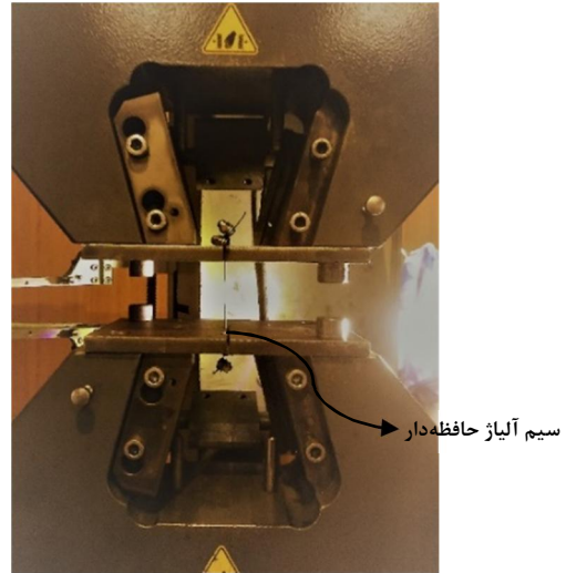
شکل ۴- کشش سیم آلیاژ در دستگاه
