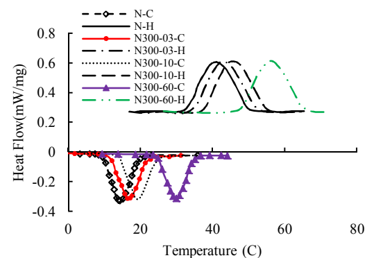
شکل ۸- نمودار شار حرارتی بر حسب دما برای درجه ۳۰۰
