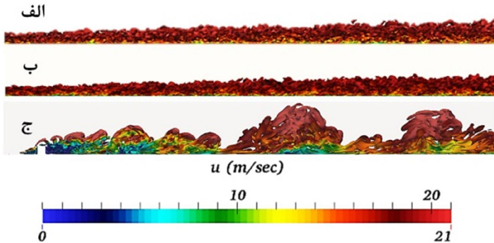
شکل ۶- کانتور معیار کیو ( Q=2 \times 10^5 )، رنگ آمیزی شده با مقادیر سرعت لحظه‌ای، الف) مدل مرز ورودی مبتنی بر حل اولیه و ب) مدل مرز ورودی لاند ج) مدل مرز ورودی سرعت یکنواخت و آشفته‌سازی توسط تریپ
