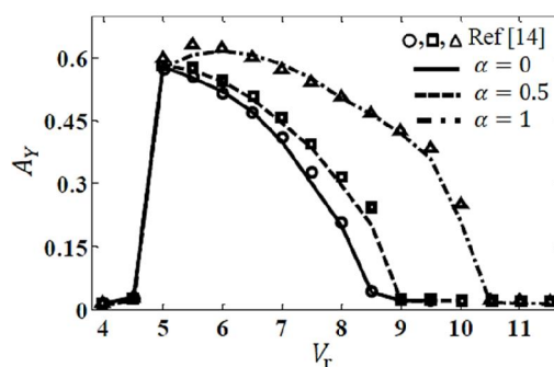
شکل ۳- دامنه پاسخ جابجایی عرضی استوانه بر حسب سرعت کاهش یافته برای استوانه مرتعش چرخان و غیر چرخان
