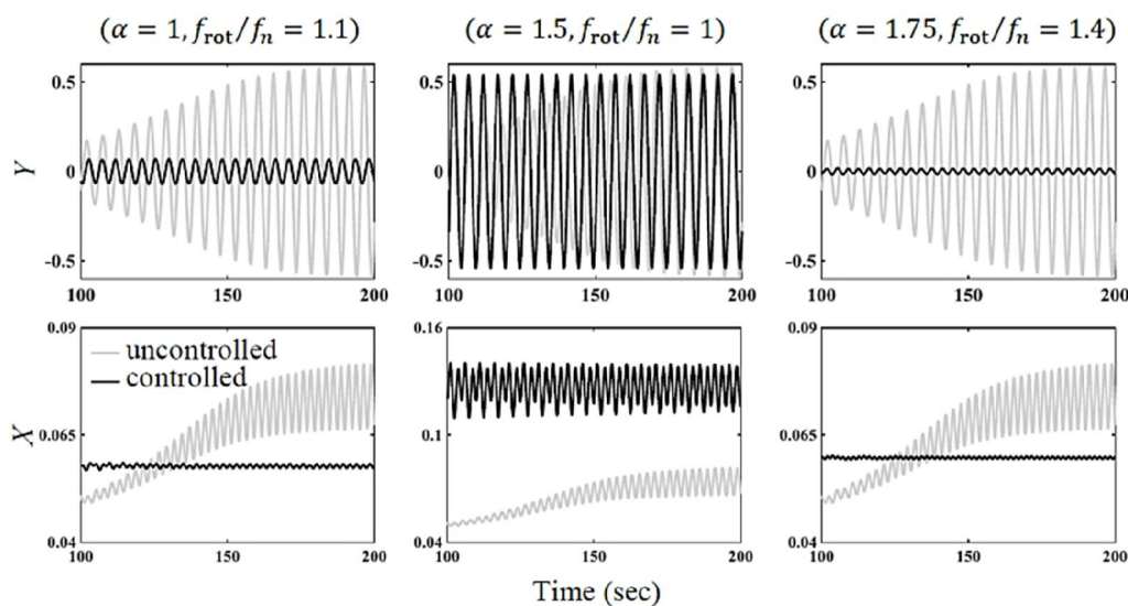
شکل ۱۲- تاریخچه زمانی جابجایی عرضی و طولی بی بعد شده استوانه در V_r = 5
