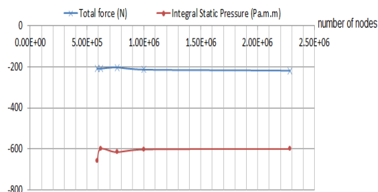
شکل ۵- مقادیر نیروی کل و مجموع فشار استاتیکی وارد بر ساختمان بر حسب تعداد گره‌ها
