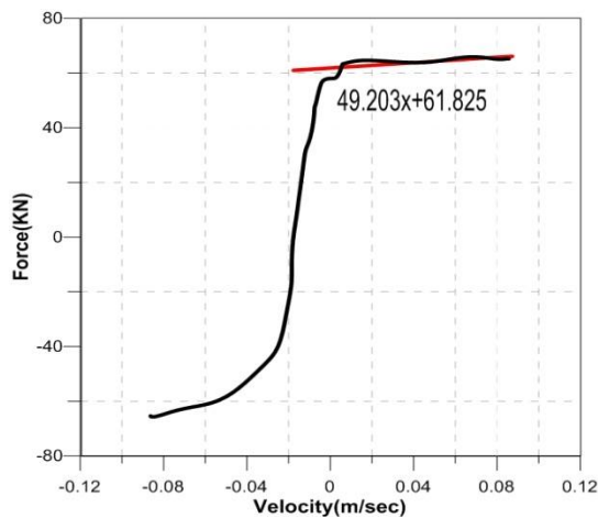
شکل ۶- مرحله بارگذاری دیاگرام "نیروی بهروز شده- سرعت" به منظور محاسبه k_x و k_\omega
