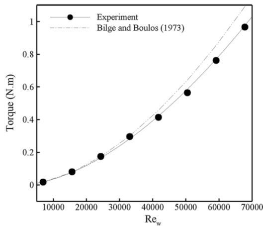
شکل ۴- اعتبارسنجی سیستم تیلور-کوئت در جریان‌های تک فاز
