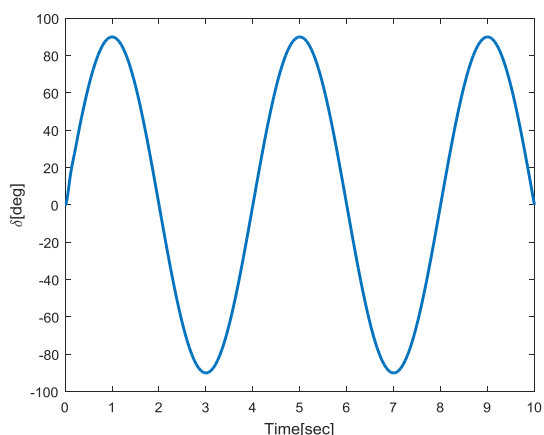
شکل ۱۸- حرکت فرمان برای آزمایش موج سینوسی
