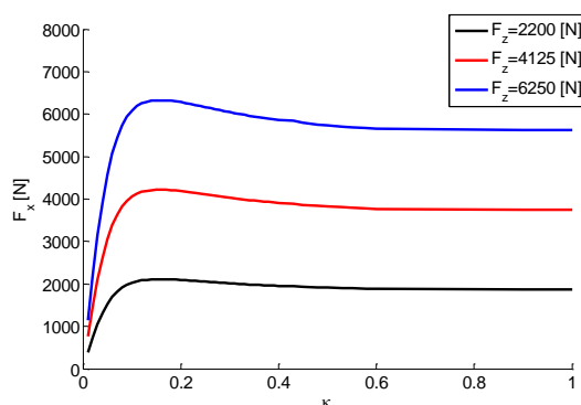
شکل ۵- نیروی طولی تاپر
