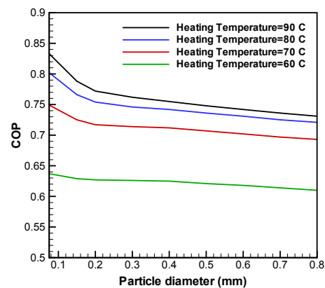
شکل ۴- مقدار ضریب عملکرد نسبت به قطر ذرات در دمای آب گرم مختلف
