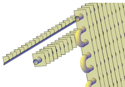
شکل ۲- مبدل حرارتی با فین‌های صفحه‌ای به عنوان بستر ماده جاذب
