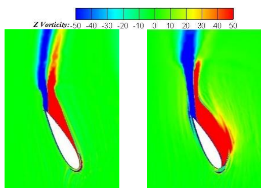
شکل ۱۵- کانتور گردابه حول ایرفویل اول مدل ترکیبی (الف) ۱ و (ب) ۳
