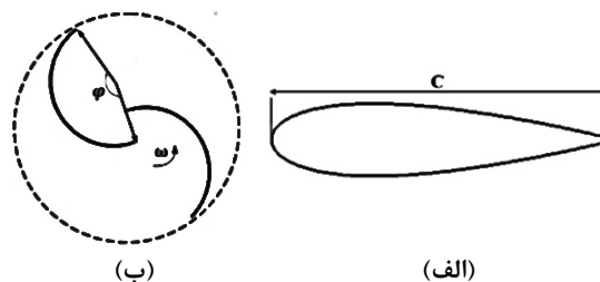
شکل ۸- نمایش پارامترهای موردبررسی، الف) طول وتر ایرفویل و ب) زاویه‌ی کمان پره‌ی ساونیوس
