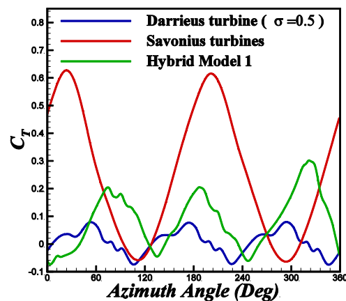
شکل ۱۰- مقایسه‌ی ضریب گشتاور توربین‌های داریوس، ساونیوس و ترکیبی در نسبت سرعت نوک (الف) ۰/۵ و (ب) ۱
