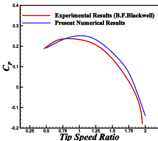
شکل ۴- مقایسه‌ی نتایج آزمایشگاهی بلک‌ول با نتایج عددی حاضر برای توربین ساوینیوس
