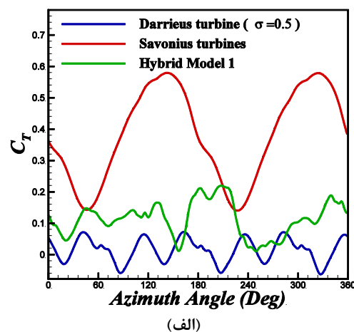
شکل ۹- مقایسه‌ی منحنی عملکرد توربین‌های داریوس، ساونیوس و ترکیبی
