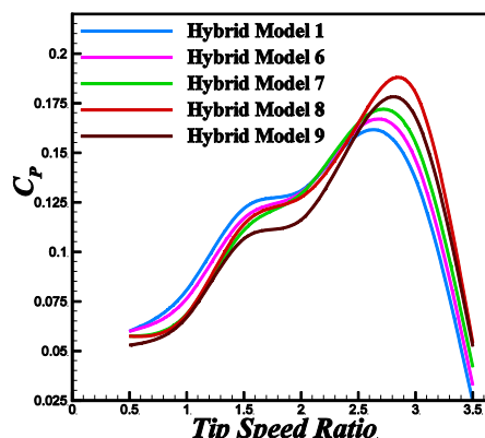
شکل ۱۶- مقایسه منحنی عملکرد مدل‌های ترکیبی ۱، ۶، ۷، ۸، ۹
