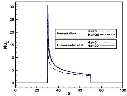
شکل ۳-ب - مقایسه تغییرات عدد ناسلت با مقادیر حاصل از کار امین الساداتی و همکاران [۳۴]، در طول دیوار ریزکانال در اعداد هارتمن مختلف برای Re=100 و \phi=0.02
