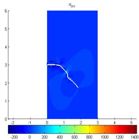
شکل ۱۷- رشد ترک لبه‌ای در شرایط مرزی متفاوت: درجات آزادی کف دامنه بسته شده‌اند
