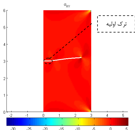
شکل ۱۵- نحوه رشد ترک لبه‌ای
