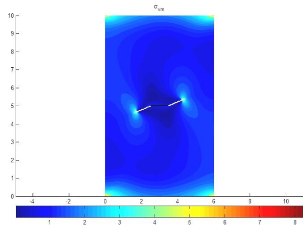
شکل ۹- اثر شرایط مرزی بر گسترش ترک افقی
