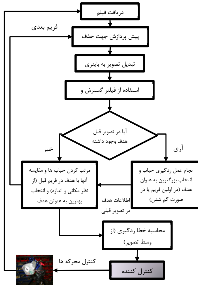
شکل ۳- الگوریتم ردگیری
