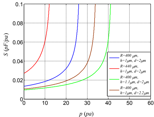
شکل ۱۱- اثر پارامترهای هندسی بر حساسیت میکرو حسگر تحت ولتاژ ۲ ولت
