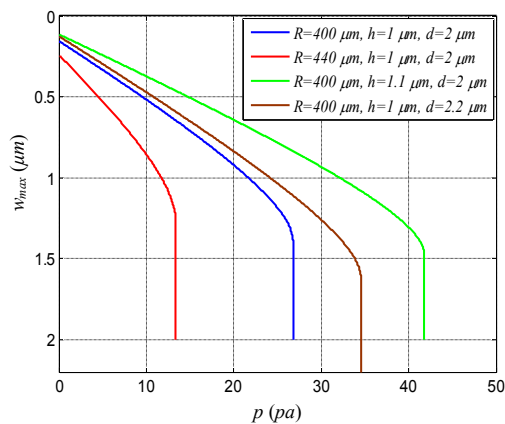
شکل ۷- اثر پارامترهای هندسی بر خیز بیشینه میکرو حسگر تحت ولتاژ ۲ ولت
