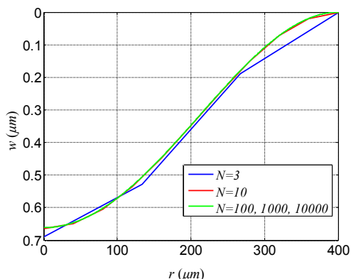
شکل ۵- خیز میکرو ورق تحت ولتاژ ۳ ولت و فشار ۵ پاسکال با در نظر گرفتن تعداد نقاط مختلف در جهت شعاع
