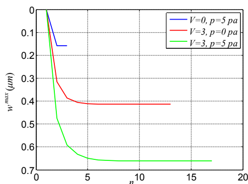
شکل ۴- همگرایی الگوریتم حل خیز استاتیکی ورق
