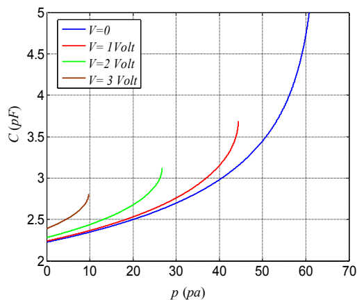
شکل ۸- ظرفیت خازنی میکرو حسگر بر حسب فشار اعمالی
