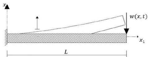
شکل ۱- فرم شماتیک جابه‌جایی خارج از صفحه میکروتیر
