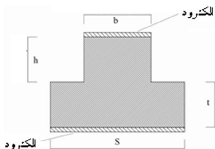
شکل ۲- پارامترهای هندسی سطح مقطع میکروتیر
