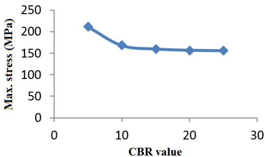
شکل ۱۰- تغییرات بیشینه تنش در صفحات ترمیم‌کننده باند فرودگاه بر حسب تغییرات شاخص خاک
