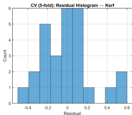
شکل ۳- هیستوگرام باقیمانده‌های پیش‌بینی مدل رگرسیون فرآیند گاوسی برای پهنای شکاف برش بر اساس اعتبارسنجی متقاطع پنج‌بخشی
