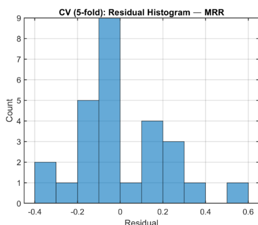
شکل ۴- هیستوگرام باقیمانده‌های پیش‌بینی مدل رگرسیون فرآیند گاوسی برای نرخ براده‌برداری بر اساس اعتبارسنجی متقاطع پنج‌بخشی
