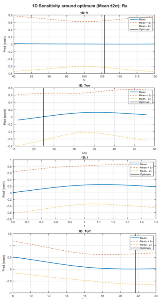
شکل ۶- آنالیز حساسیت یک‌بعدی زبری سطح اطراف نقطه بهینه با استفاده از مدل رگرسیون فرآیند گاوسی (میانگین پیش‌بینی و باندهای 2\pm\sigma )
