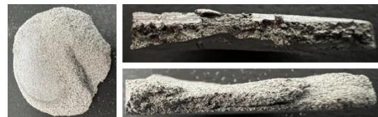
شکل ۱- تصاویر نمونه‌های اولیه ساخته شده با کیفیت غیرقابل قبول.
