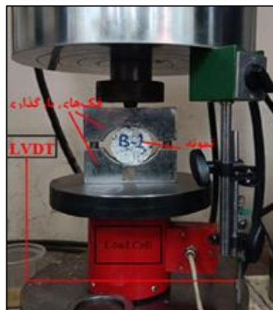
شکل ۷- دستگاه آزمایش کشش برزیلی
