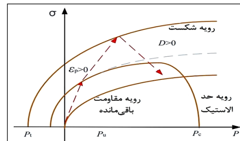
شکل ۴- نمای مدل مقاومتی مدل ساختاری RHT [۱۱]
