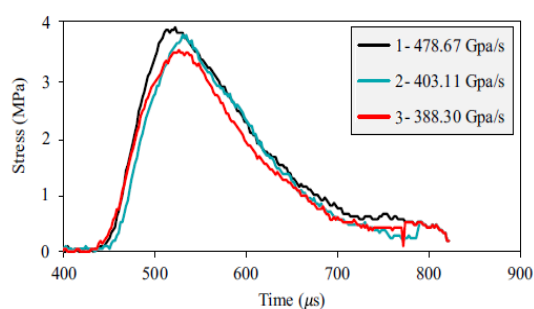
شکل ۱۰- تحلیل موج عبوری دینامیکی سه آزمایش هایکینسون برزلی
