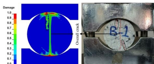
شکل ۲۳- مقایسه الگوی شکست در آزمایش کشش برزیلی و شبیه‌سازی عددی
