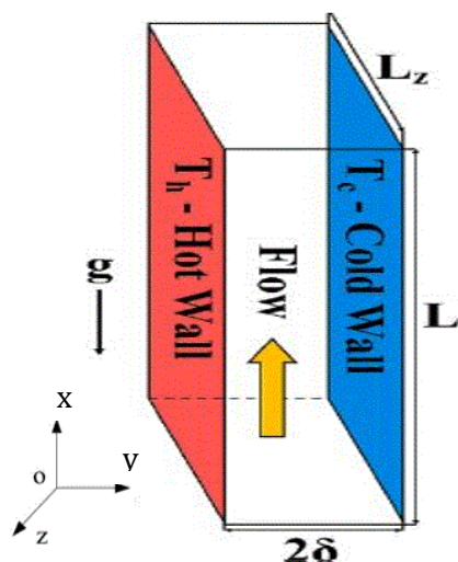
شکل ۱- دستگاه مختصات و هندسه جریان
