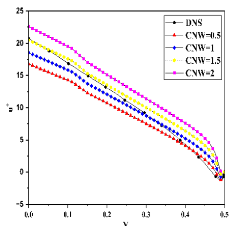
شکل ۲۳- سرعت بدون بُعد حاصل از نتایج DNS و GEKO در سمت جریان مخالف برای Ri=1 با مقادیر cnw مختلف
