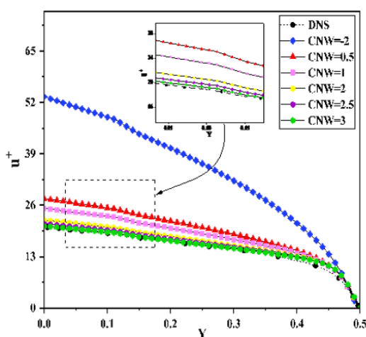
شکل ۱۷- سرعت بدون بُعد حاصل از نتایج DNS و GEKO در سمت جریان مخالف برای Ri=0.25 با مقادیر مختلف cnw
