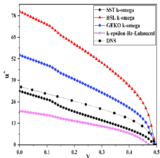
شکل ۱۱- سرعت بدون بُعد حاصل از نتایج DNS و RANS در سمت جریان مخالف برای Ri=0.5
