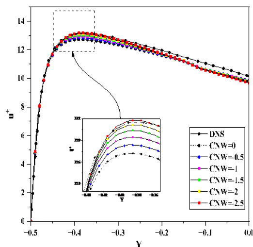
شکل ۱۶- سرعت بدون بُعد حاصل از نتایج DNS و GEKO در سمت جریان همسو برای Ri=0.25 با مقادیر مختلف cnw
