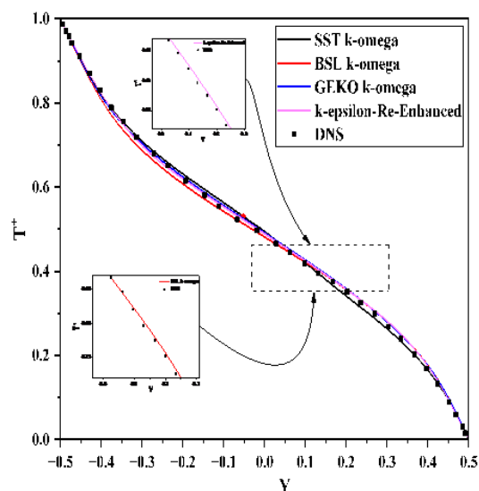
شکل ۷- دمای بدون بعد حاصل از نتایج DNS و RANS در محدوده کل جریان برای Ri=0.25
