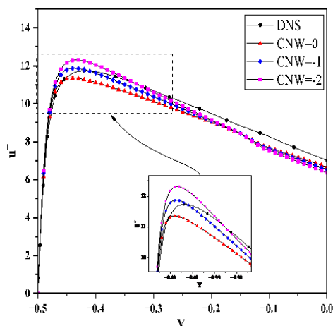
شکل ۲۲- سرعت بدون بُعد حاصل از نتایج DNS و GEKO در سمت جریان همسو برای Ri=1 با مقادیر cnw مختلف
