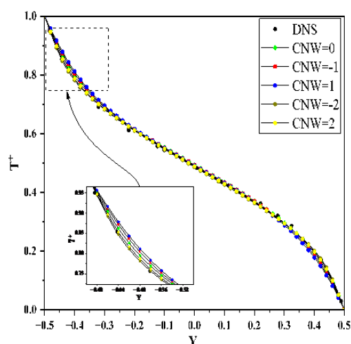
شکل ۲۱- دمای بدون بُعد حاصل از نتایج DNS و RANS در محدوده کل جریان برای Ri=0.5 با مقادیر cnw مختلف
