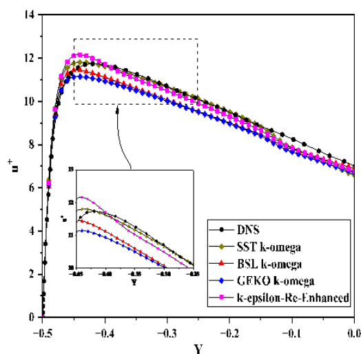
شکل ۱۶- سرعت بدون بُعد حاصل از نتایج DNS و RANS در سمت جریان همسو برای Ri=1
