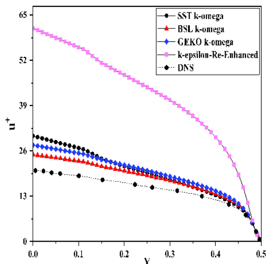
شکل ۶- سرعت بدون بُعد حاصل از نتایج DNS و RANS در سمت جریان مخالف برای Ri=0.25
