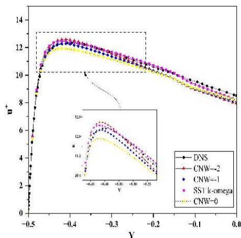
شکل ۱۹- سرعت بدون بُعد حاصل از نتایج DNS و GEKO در سمت جریان همسو برای Ri=0.5 با مقادیر مختلف cnw
