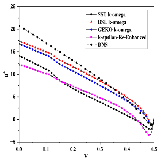
شکل ۱۴- سرعت بدون بُعد حاصل از نتایج DNS و RANS در سمت جریان مخالف برای Ri=1
