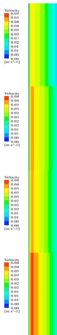
شکل ۸- کانتور سرعت برای ۴ مدل توربولانسی به ترتیب SST k- \omega ، BSL k- \omega ، GEKO k- \omega ، k- \epsilon Re-Enhanced عدد Ri=0.25
