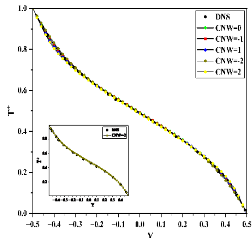
شکل ۱۸- دمای بدون بُعد حاصل از نتایج DNS و RANS در محدوده کل جریان برای Ri=0.25 با مقادیر مختلف cnw
