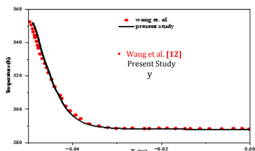
شکل ۴- نمودار تغییرات دما در مقطع x=5 m جهت اعتبارسنجی با مطالعه پوچاری و همکاران [۲۹]
