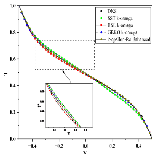
شکل ۱۲- دمای بدون بُعد حاصل از نتایج DNS و RANS در محدوده کل جریان برای Ri=0.5
