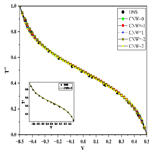
شکل ۲۴- دمای بدون بُعد حاصل از نتایج DNS و RANS در محدوده کل جریان برای Ri=1 با مقادیر مختلف cnw
