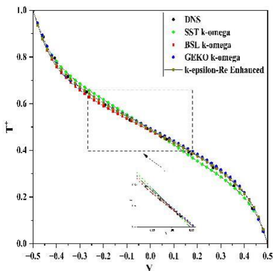
شکل ۱۵- دمای بدون بُعد حاصل از نتایج DNS و RANS در محدوده کل جریان برای Ri=1
