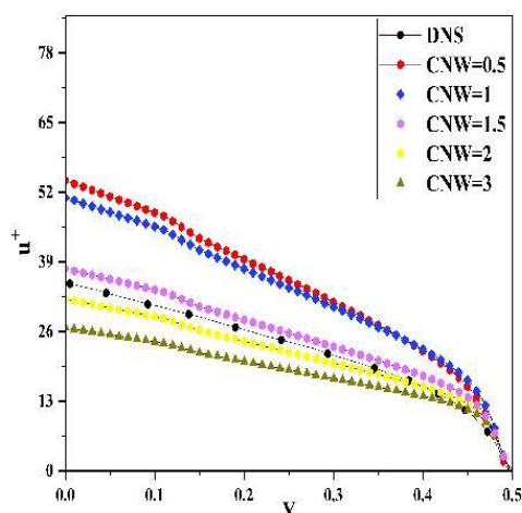
شکل ۲۰- سرعت بدون بُعد حاصل از نتایج DNS و GEKO در سمت جریان مخالف برای Ri=0.5 با مقادیر مختلف cnw
