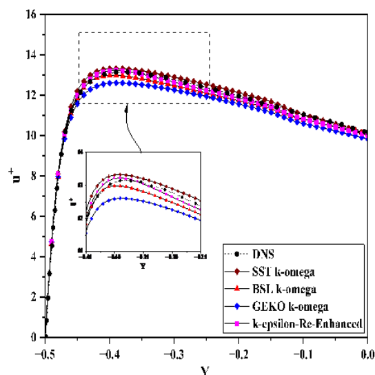
شکل ۵- سرعت بدون بُعد حاصل از نتایج DNS و RANS در سمت جریان همسو برای Ri=0.25
