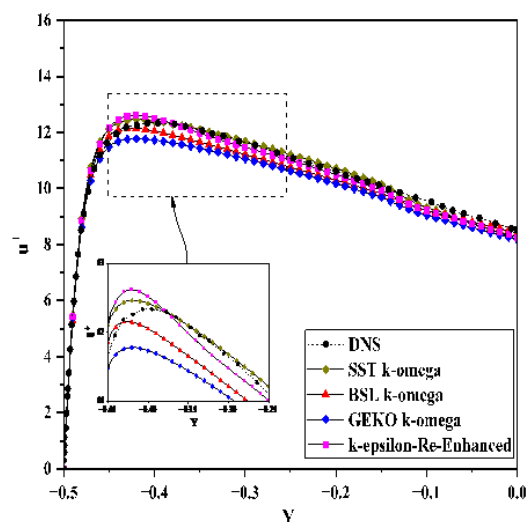
شکل ۱۰- سرعت بدون بُعد حاصل از نتایج DNS و RANS در سمت جریان همسو برای Ri=0.5
