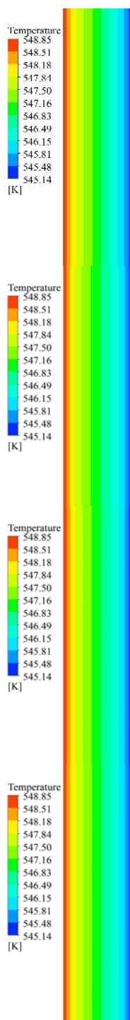
شکل ۹- کانتور دما برای ۴ مدل توربولانسی به ترتیب SST k- \omega , k- \epsilon Re-Enhanced, BSL k- \omega , GEKO k- \omega عدد Ri=0.25
