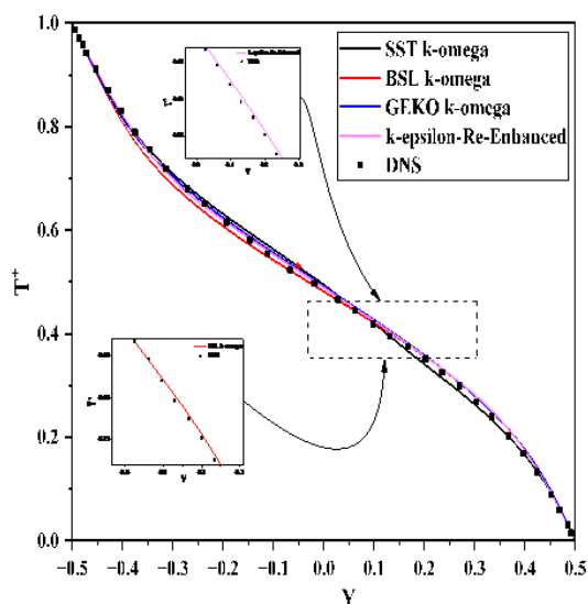
شکل ۷- دمای بدون بعد حاصل از نتایج DNS و RANS در محدوده کل جریان برای Ri=0.25
