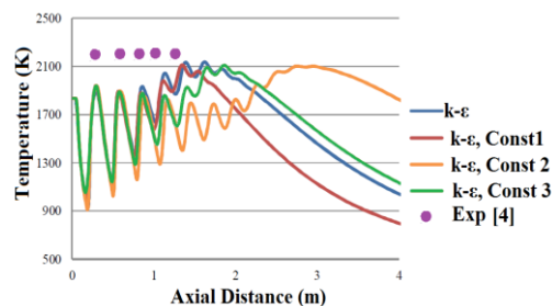
شکل ۱۰- مقایسه نتایج مدل k-\epsilon با ثابت‌های مختلف
