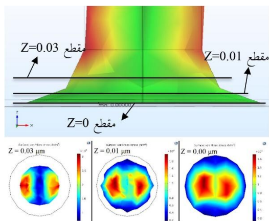
شکل ۸- بالا) محل برش های پایه‌ی مژک در ارتفاع‌های ۰/۰۳، ۰/۰۱ و ۰/۰۰۱ و صفر میکرومتر که با خط‌های تیره نشان داده شده‌اند. پایین) میدان تنش در مقاطع مژک در ارتفاع‌های ۰/۰۳، ۰/۰۱ و صفر میکرومتر به ترتیب از چپ به راست در مدل تیر یک‌سردگیر (اتصال کاملاً مقید)
