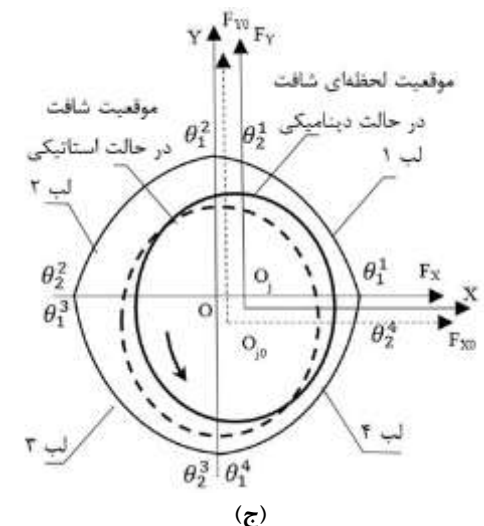
شکل ۱- هندسه یاتاقان‌های غیرمدور (الف) دویل، (ب) سه لب و (ج) چهار لب
