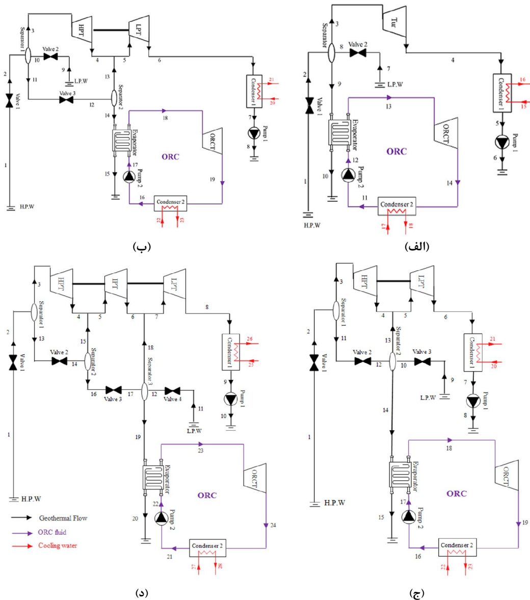
شکل ۱- شماتیک چرخه‌های ترکیبی جدید الف) تبخیر تک مرحله‌ای-باینری، ب) تبخیر دو مرحله‌ای نوع اول-باینری، ج) تبخیر دو مرحله‌ای نوع دوم-باینری و د) تبخیر سه مرحله‌ای-باینری
