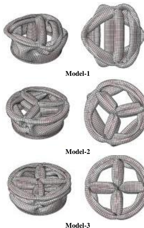
شکل ۲۱- اثر تقویت‌کننده‌های چند سلولی بر نحوه فروریزش پوسته‌های استوانه‌ای برنجی
