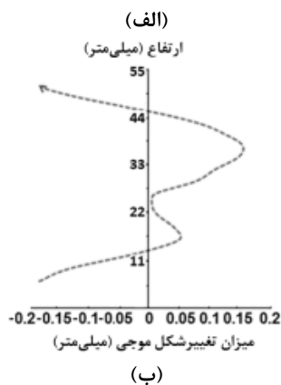
شکل ۱- الف) گرادیان ضخامت دیواره و ب) میزان برآمدگی سطح پوسته‌ی استوانه‌ای برنجی
