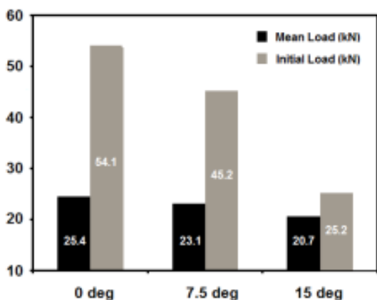
شکل ۱۹- اثر زاویه‌ی نیم‌رأس بر نیروی اولیه و متوسط نیروی فروریزش پوسته‌ی استوانه‌ای برنجی تحت بارگذاری محوری
