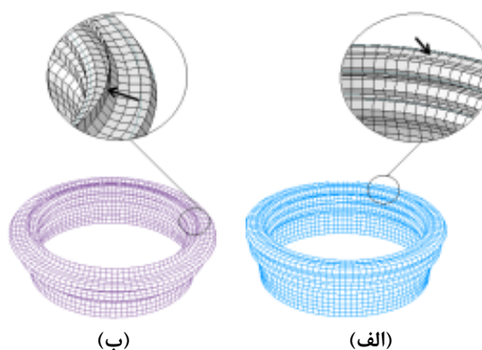
شکل ۱۷- مقایسه‌ی نحوه‌ی فروریزش پوسته‌های استوانه‌ای برنجی تحت شرایط مرزی؛ الف) یک‌سری‌دار و ب) دوسری‌دار
