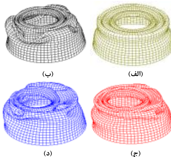
شکل ۲۴- اثر زاویه‌ی برخورد بر نحوه‌ی فروریزش پوسته‌های مخروطی با زاویه نیم‌رأس ۱۵ درجه با زاویه برخورد الف) صفر درجه، ب) ۵ درجه، ج) ۱۰ درجه و د) ۱۵ درجه
