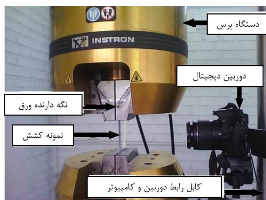
شکل ۳- طرح آزمون کشش تک‌محوری و موقعیت اجزاء
