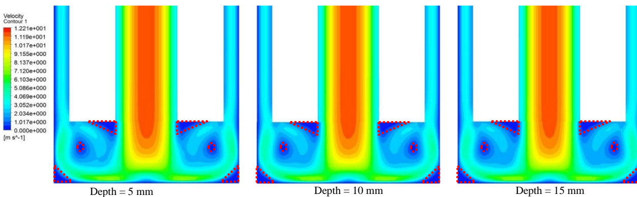
شکل ۸- کانتورهای سرعت
