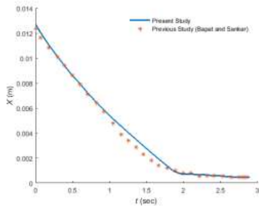
شکل ۸- ارزیابی میراگر ضربه‌ای تک‌جرمی با پژوهش بابت و سانکر [۸]
