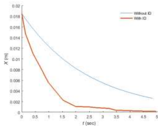
شکل ۷- دامنه ارتعاشات سیستم با و بدون میراگر ضربه‌ای سه‌جرمی
