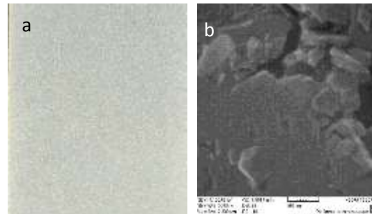
شکل ۲- (a) تصویر واقعی از نمونه سندبلاست شده و (b) تصویر با بزرگنمایی ۵۰۰۰۰ برابر از نمونه اول
