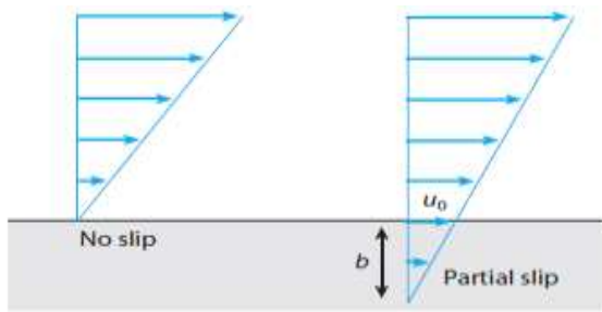
شکل ۱- طول لغزش b
