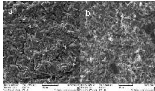
شکل ۳- (a) تصویر نمونه آماده شده بعد از فرایند جوشش و (b) تصویر نمونه آماده شده بعد از فرایند آبرگریزی
