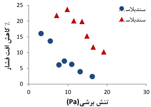
شکل ۱۰- کاهش افت فشار در کانال ۱ و ۲
