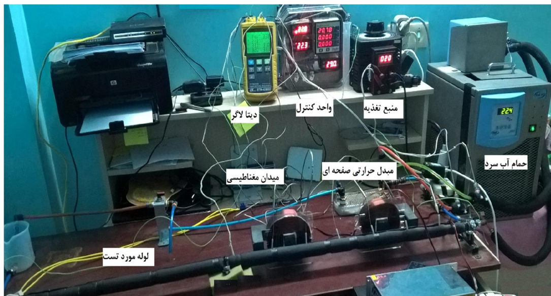
شکل ۲- تصویر دستگاه آزمایش و قسمتهای مختلف آن
