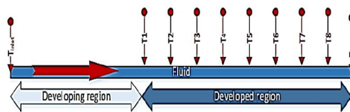
شکل ۴- موقعیت قرارگیری ترموکوپلها روی سطح لوله
